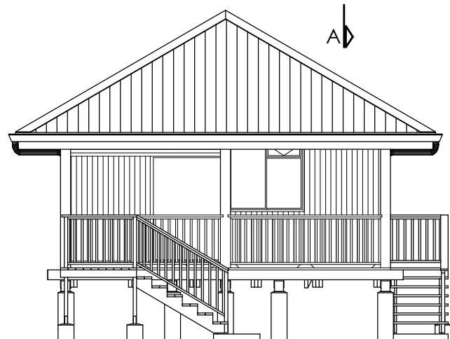
Elévation avant
