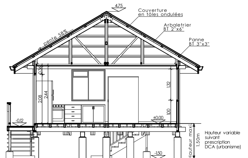
Coupe AA
