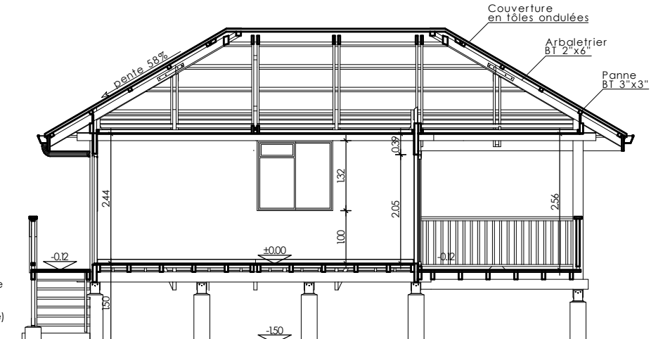
Coupe BB
