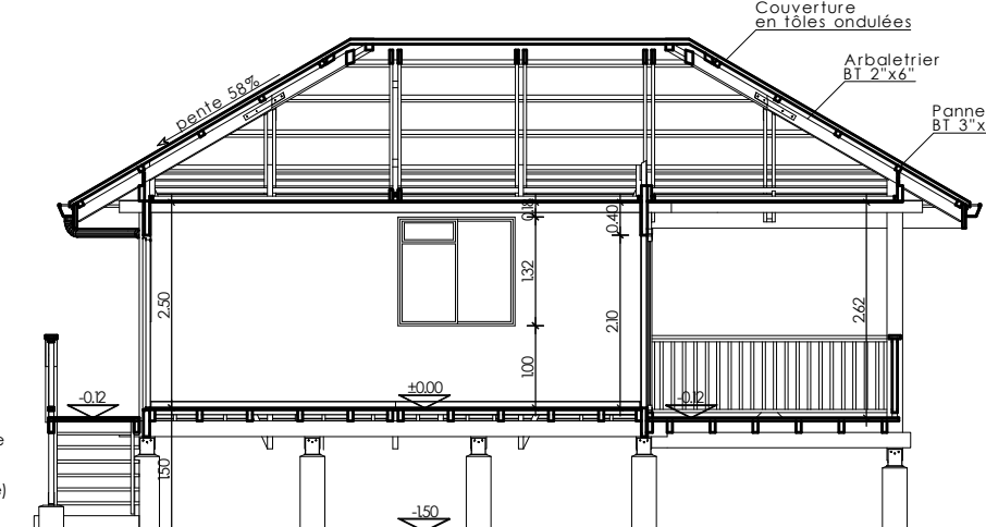
Coupe BB
