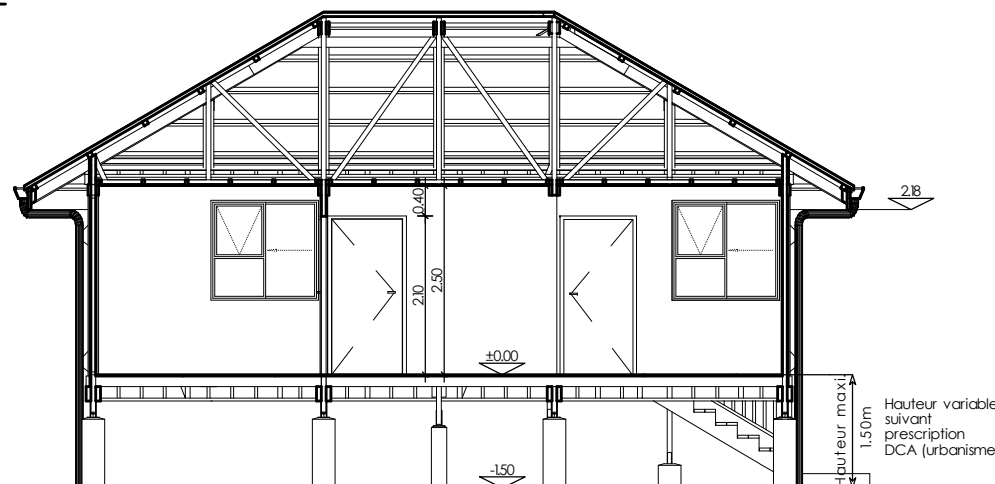
Coupe AA
