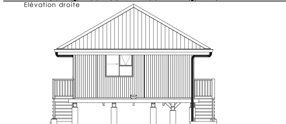
Elévation gauche
